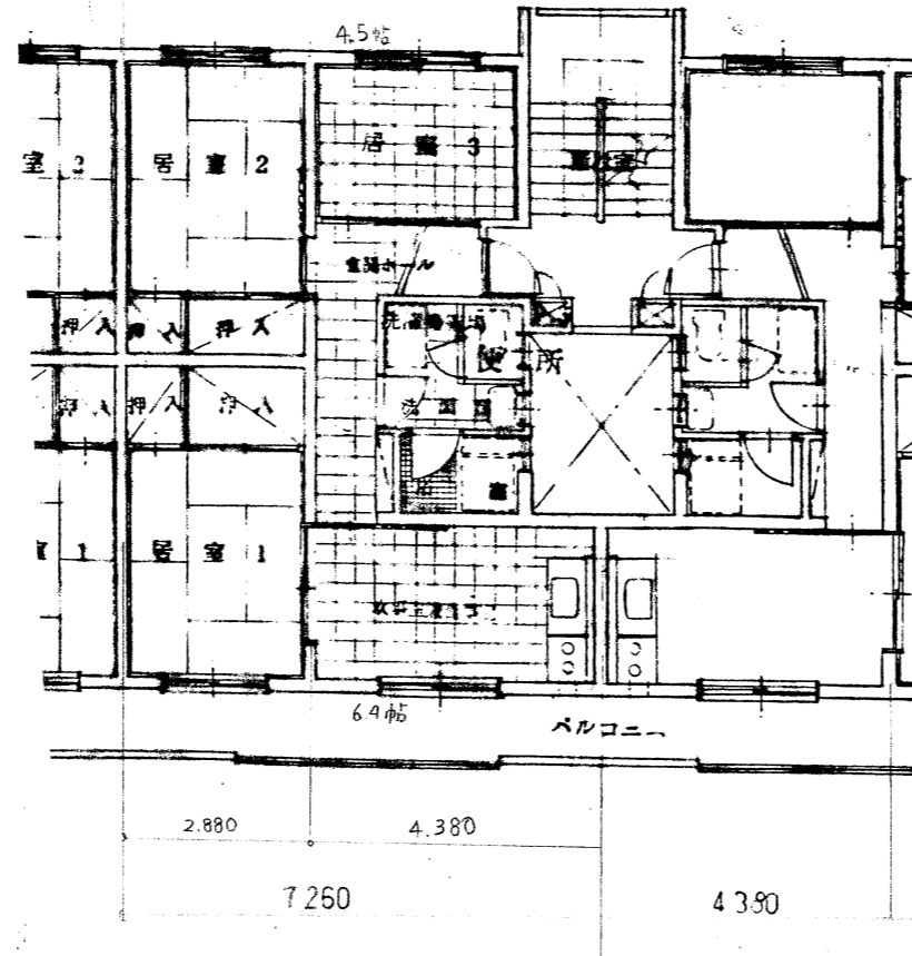
北側立面図 (西郷団地B棟-16戸)
