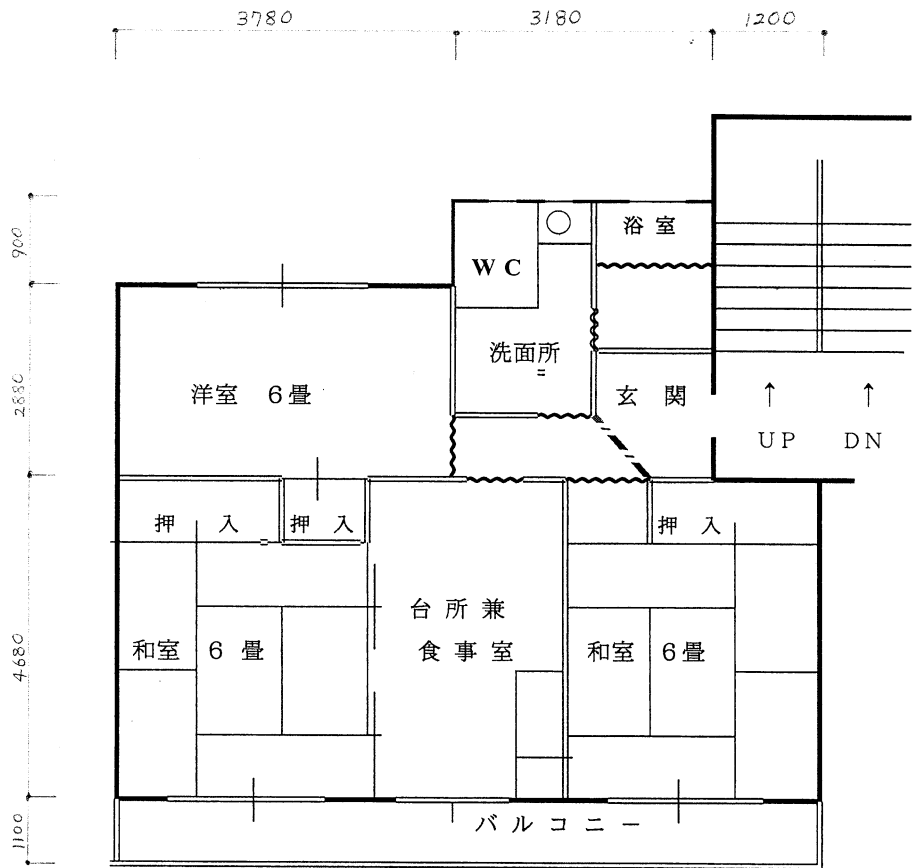
桜馬場団地 A棟 平面図(一般 - 61.09㎡) ※実際の住戸とは若干異なることがあります。
