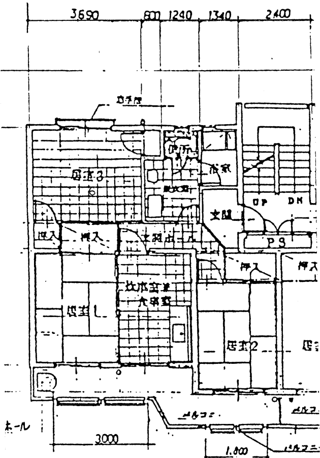
松山団地 A棟 平面図（一般 - 61.05㎡）
