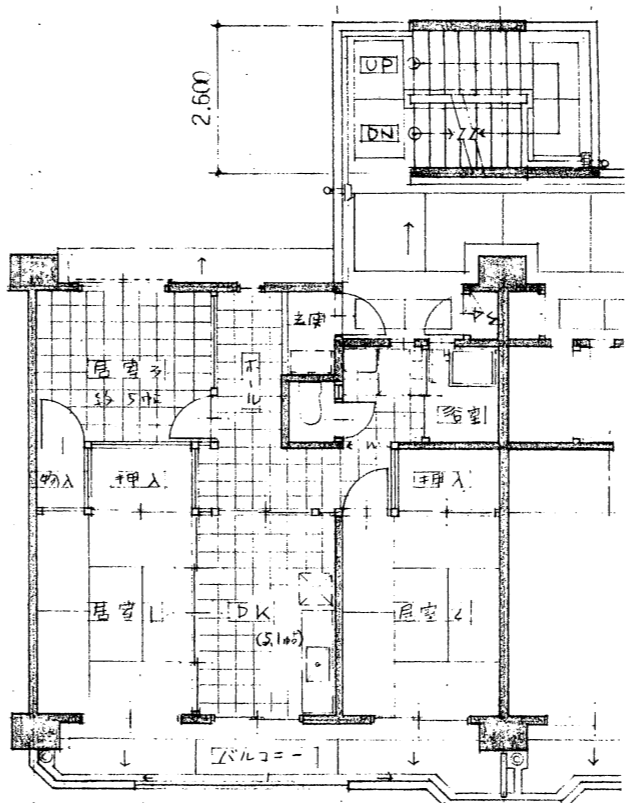
幸町団地 A棟 平面図 (一般 - 60.81㎡)
