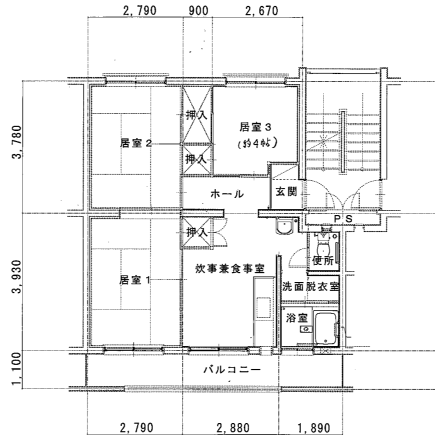
平面図
